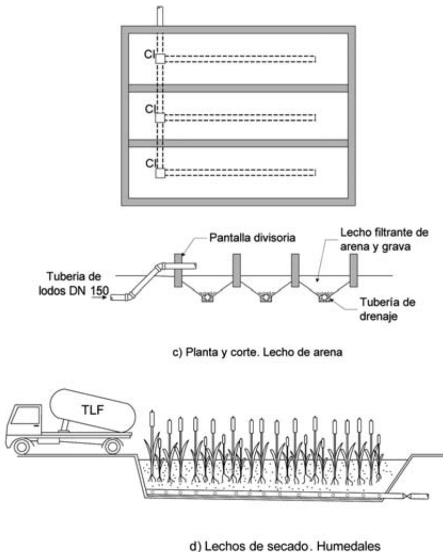
Fig. 5. Detalles constructivos. Lechos de secado de lodos
