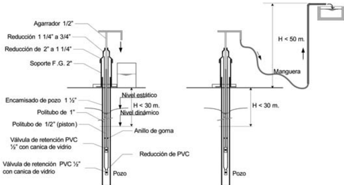
Fig. 1 Bomba manual Directa
