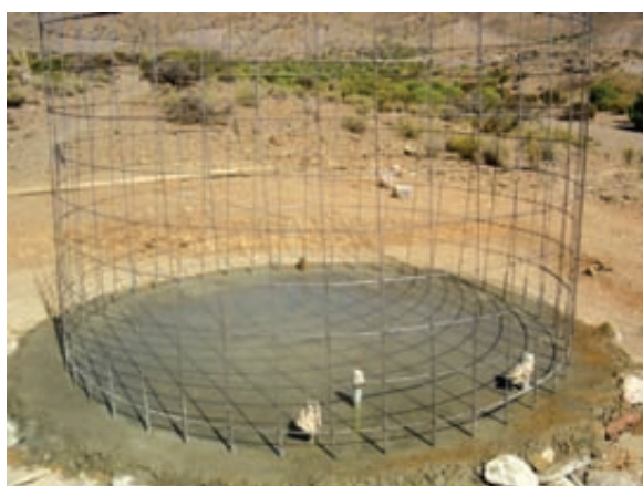
Foto 1.3. Armadura Vertical
