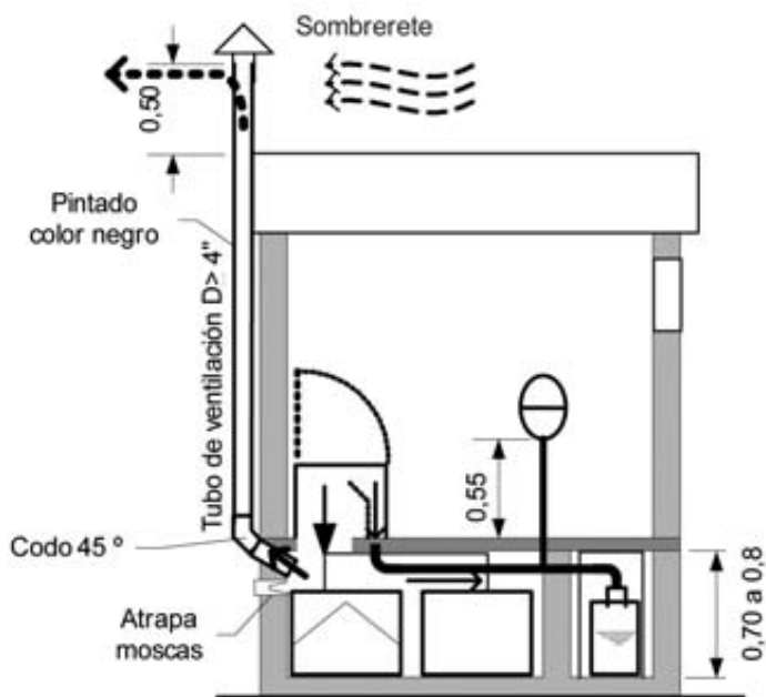
Fig. 3. Corte 2
